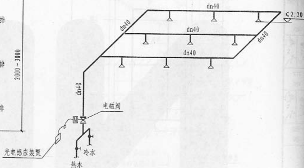
系统图
