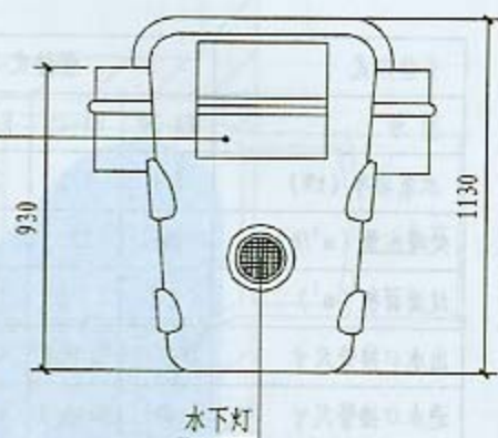
立面图
