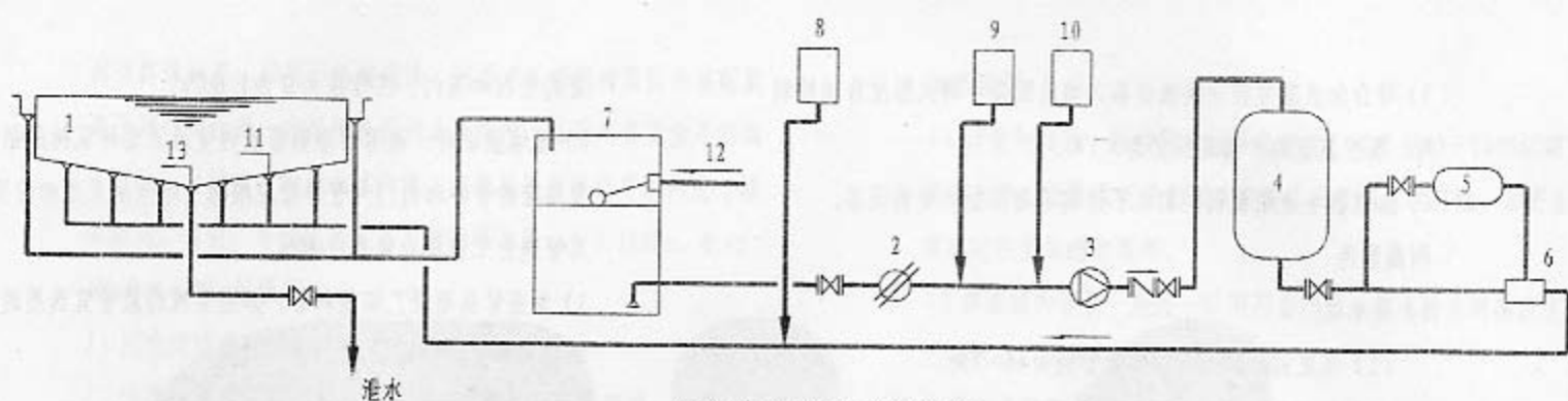
逆流式循环方式原理图
