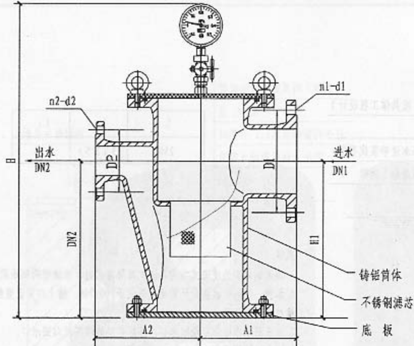
K型毛发聚集器外形图
