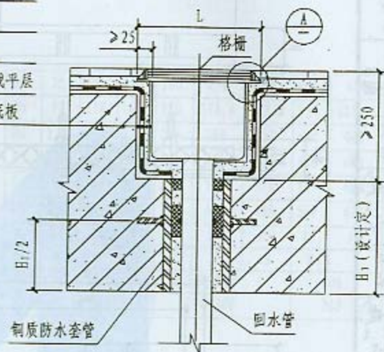
回水口安装图
