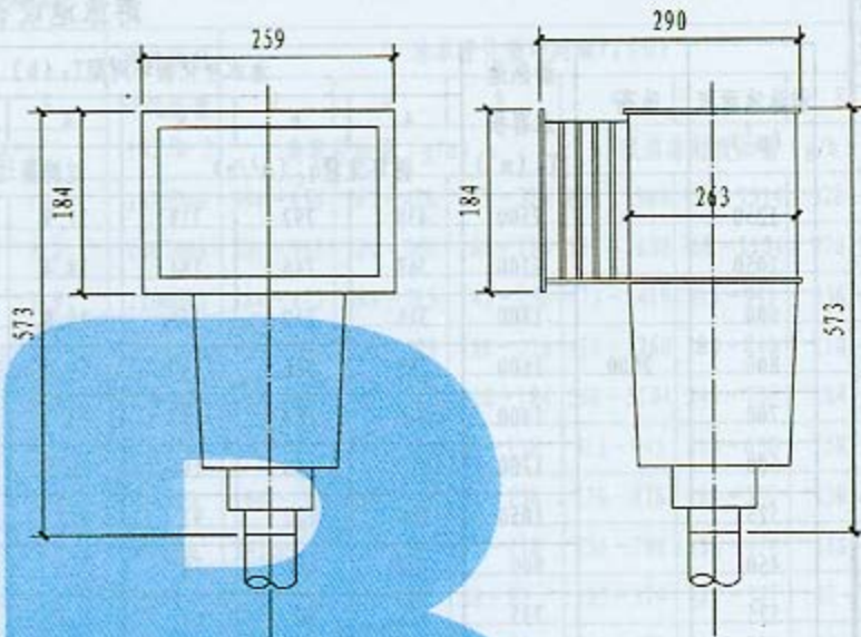
水面撇渣器
