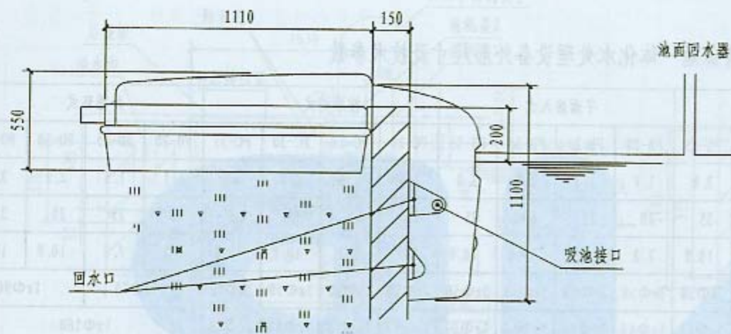
A-A剖面图
