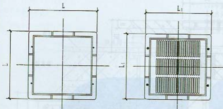
回水口盖板
