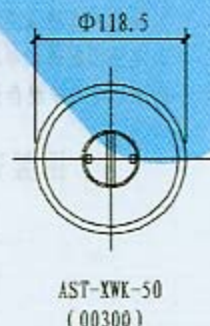
吸污接口平面图
