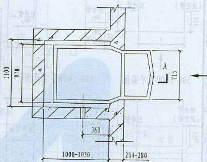
平面图
